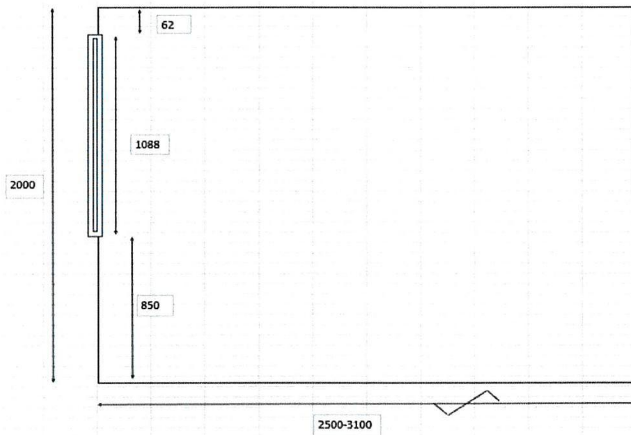
Eksempel oppriss soverom/stue
